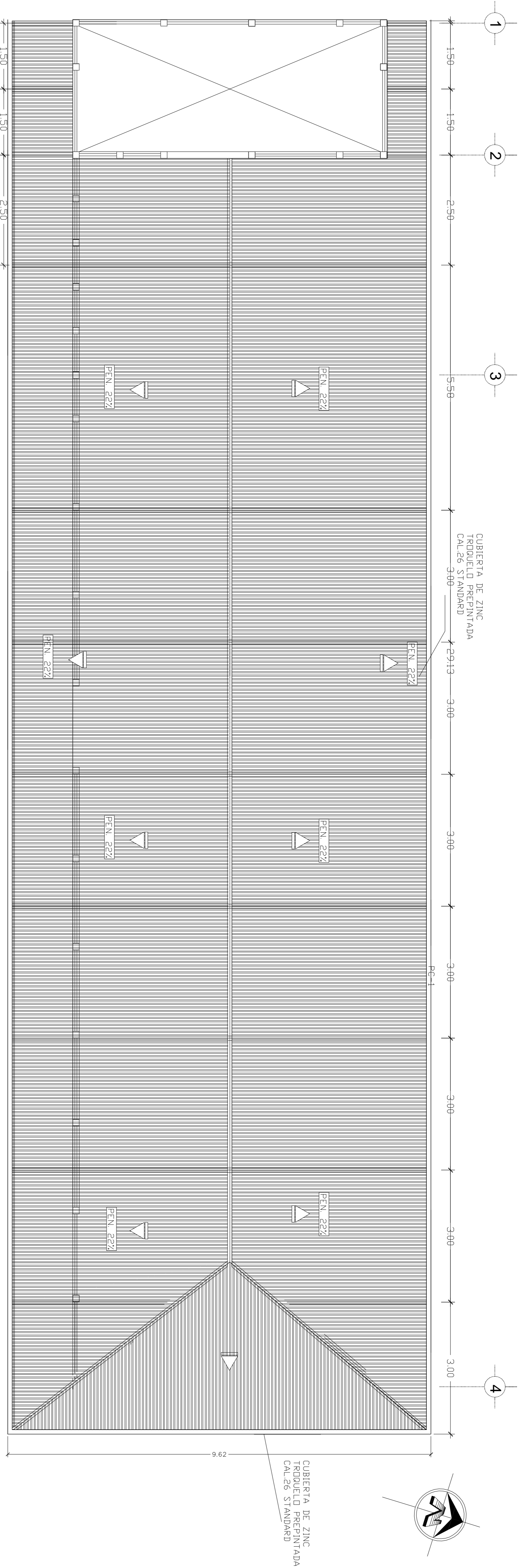
PLANTA ARQUITECTONICA DE TECHO ESCALA: 1:80
